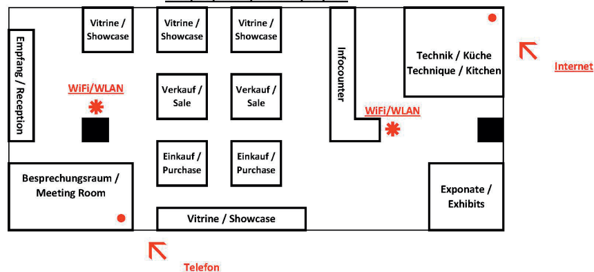
Beispielplan | Example plan
