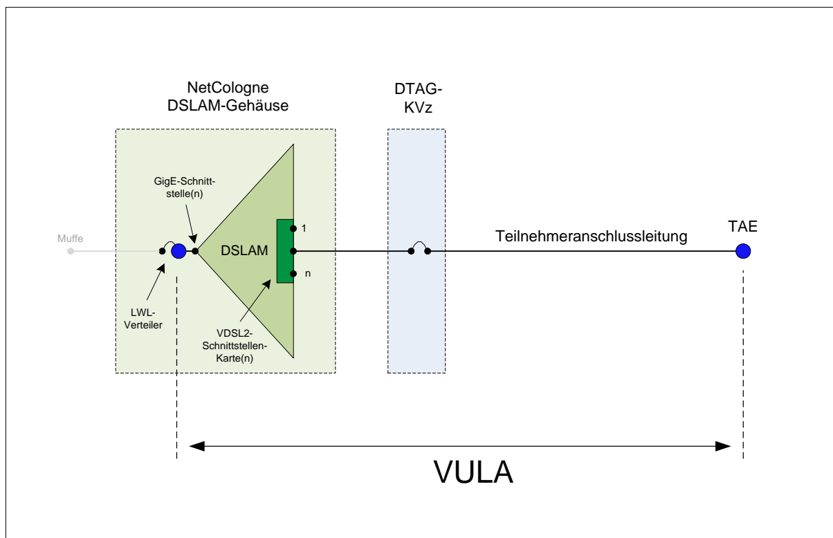
Abbildung 1 - Leistungsabgrenzung VULA
