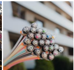
Haupttrasse (Microrohre)
